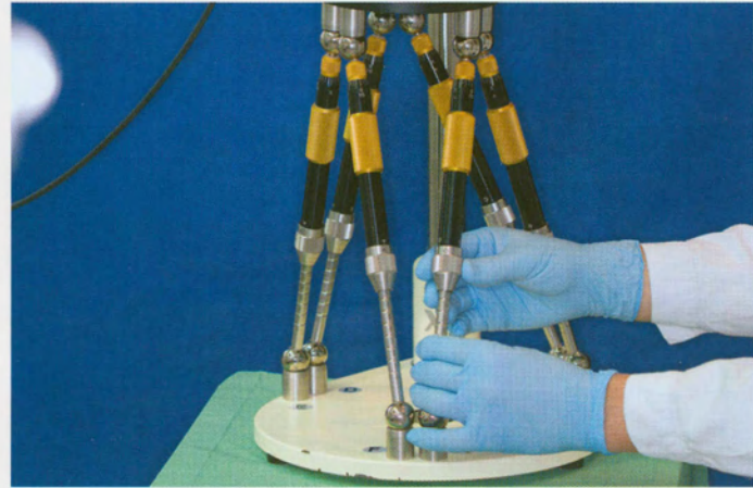
Abb. 37 Einstellung der Beinlängen vom Positionierer
