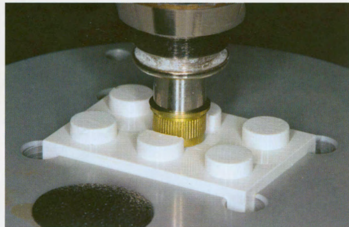
Abb. 39 Kalibrierung des Tiefenanschlags vor dem Setzen der Führungshülsen
