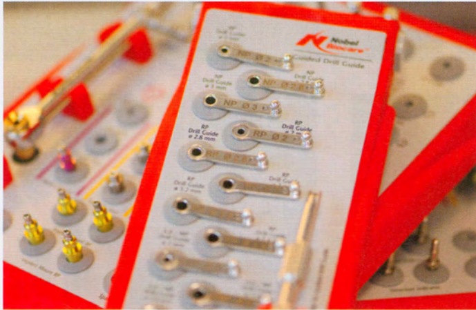
Abb. 18 und 19 Das verwendete Bohrer-Hülensystem und die fertig inserierten Implantate
